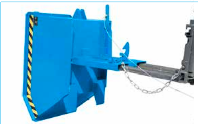
Abkippmechanismus
