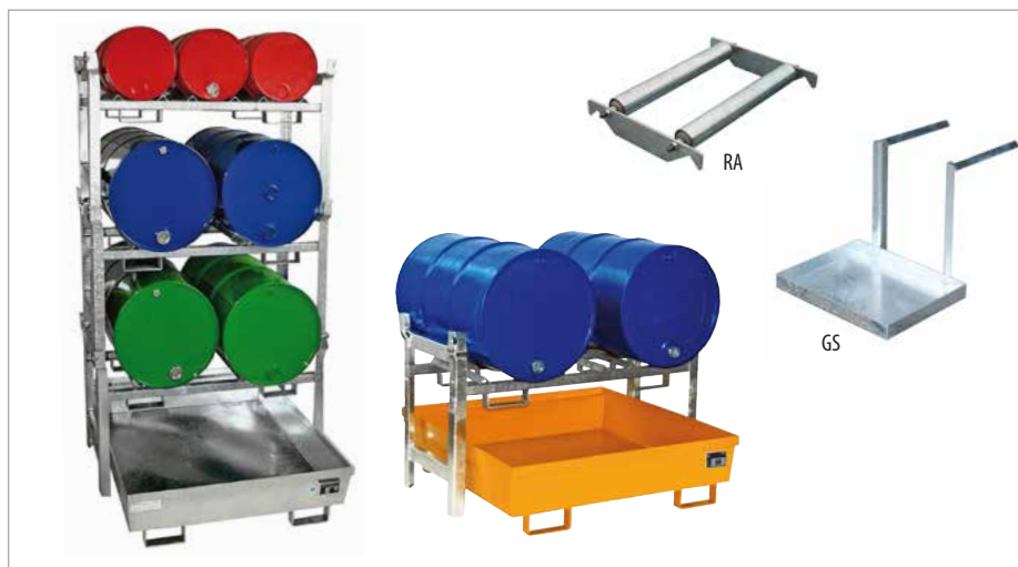
Kombinationsbeispiele: FRA-2 + 2x FR-2 + FR-3
