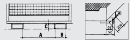
Einfahrtaschen-Innenmaße (mm)
