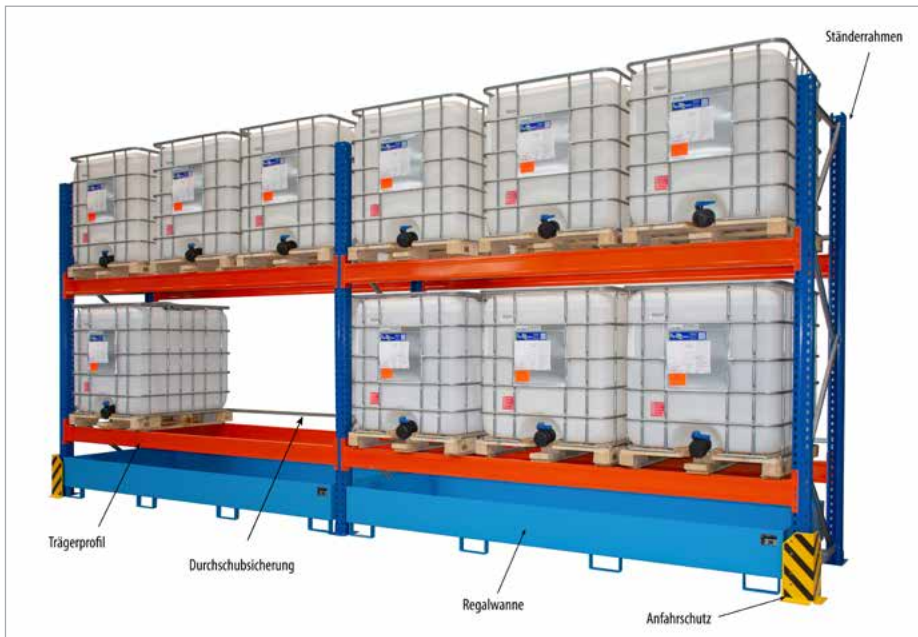
Grundregal UR-G 3300 und Anbauregal UR-A 3300 mit 2x RW 3300-3, Anfahrerschutz (Zubehör)
