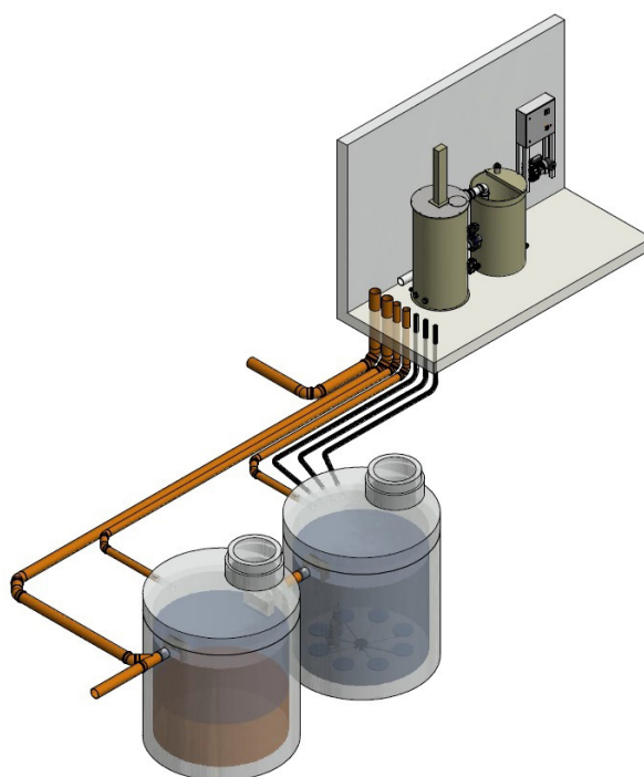
Principe de fonctionnement de l'installation BioSimplex® Ciron, installation enterrée
