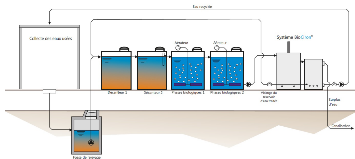
BioSimplex® Ciron - schéma d'une installation hors sol
