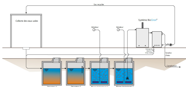
BioSimplex® Ciron - schéma d'une installation enterrée
