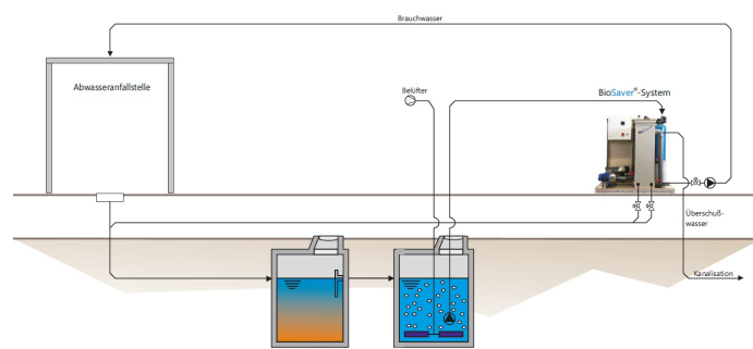
BioSimplex® Saver - Prinzipskizze unterirdisch
