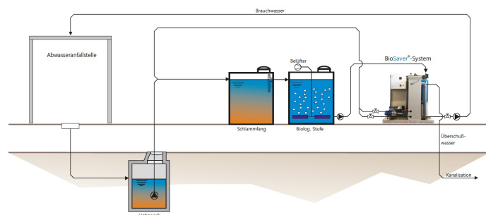
BioSimplex® Saver - Prinzipskizze oberirdisch
