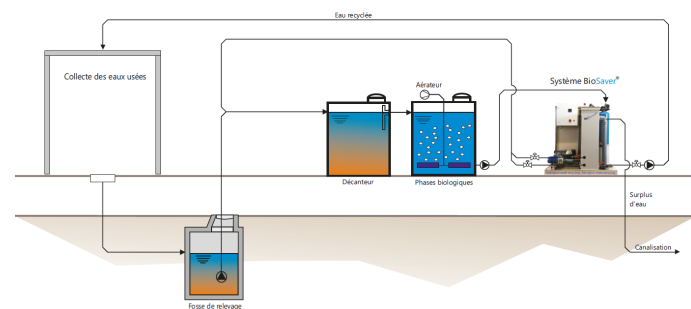
BioSimplex® Saver - schéma d'une installation hors sol
