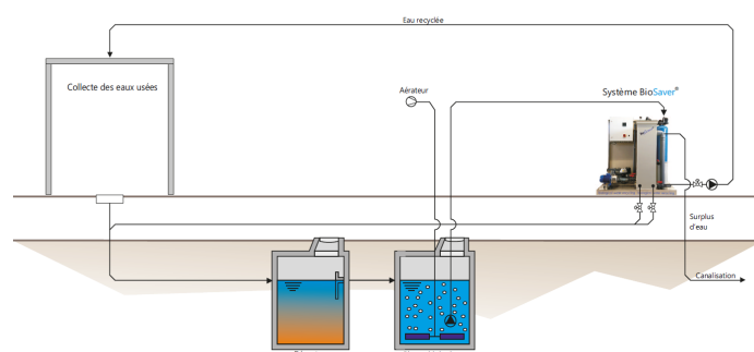
BioSimplex® Saver - schéma d'une installation enterrée
